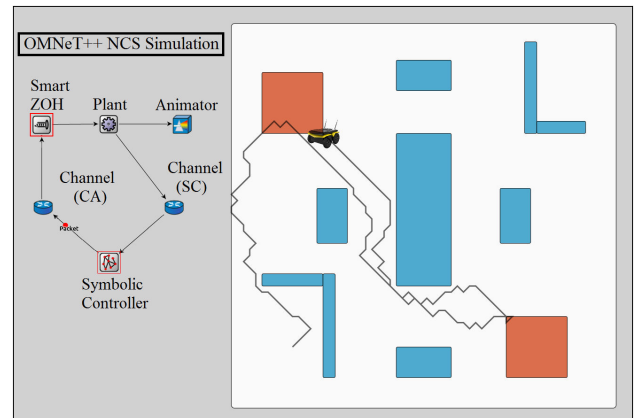
(b) OMNeT++
